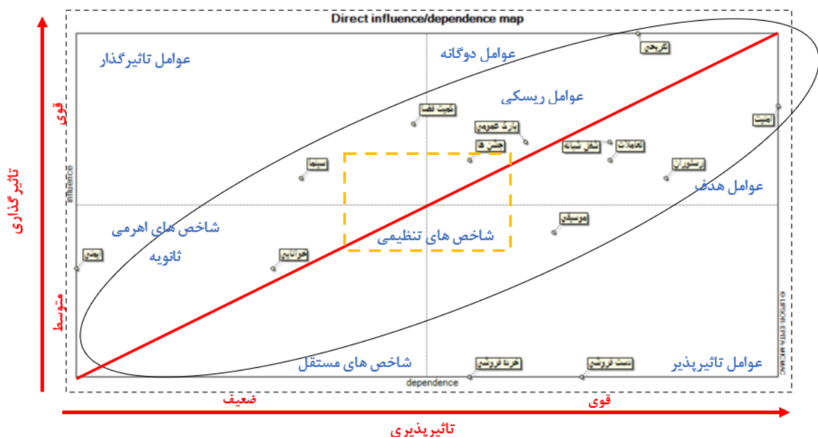
شکل ۲. پراکنش شاخص‌ها در پلان تأثیرگذاری و تأثیرپذیری مستقیم برگرفته از نرم‌افزار میک‌مک
